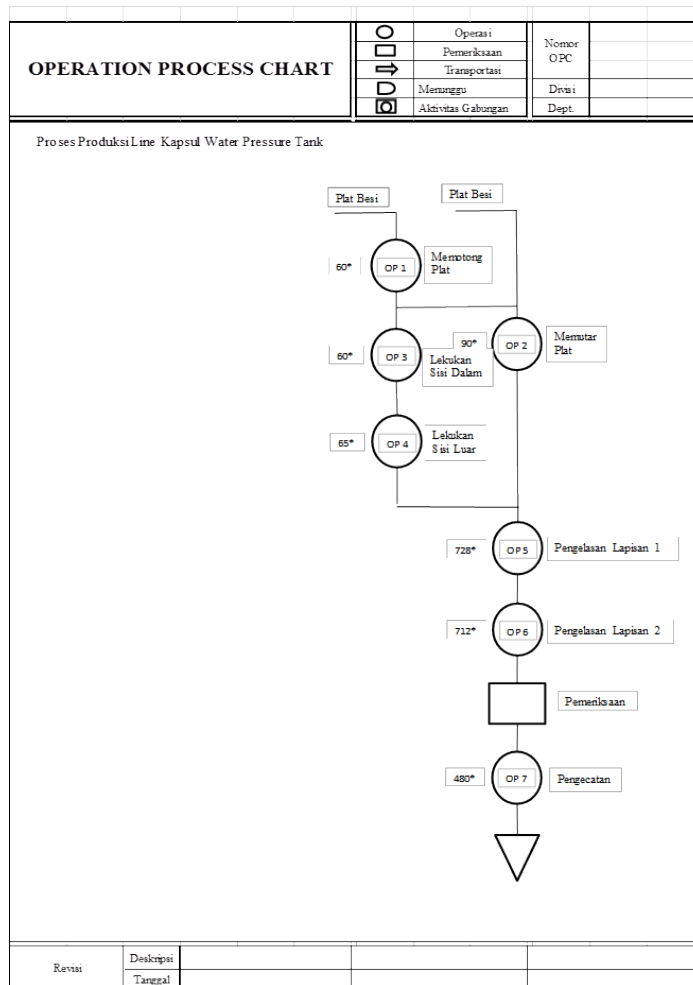
Gambar 3. OPC Proses Produksi Water Pressure Tank
