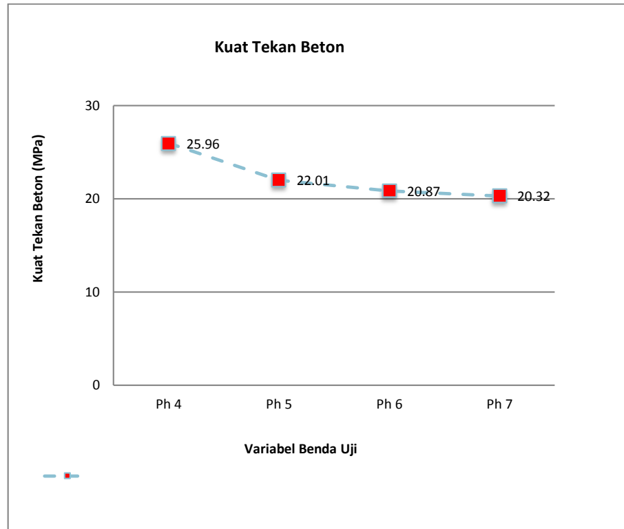
Gambar 1. Grafik Perbandingan Kuat Tekan
