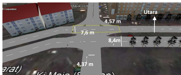
Gambar 4. Gambar Geometri Jalan
